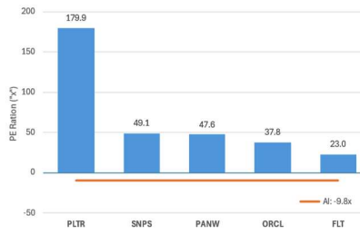
PE ratio
